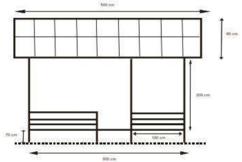
Tampak Depan
