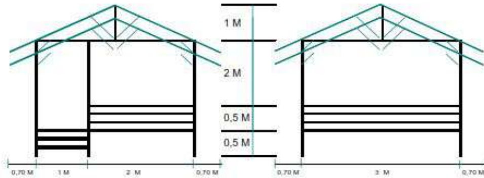
Tampak Depan
