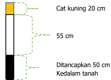
Gambar 4.1. Patok Larikan
